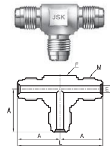
Union Tee (TUT)
