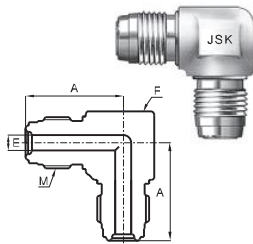
Union Elbow (TUE)
